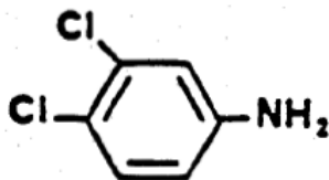
3,4-dichloroaminobenzene
