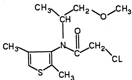
SAN 582H
