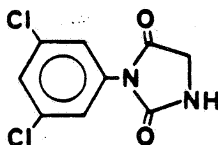
1-(3,5-Dichlorophenyl)-3-hydantoin (RP-25040)
