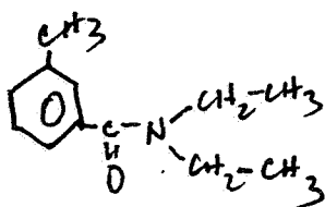
DEET
