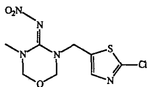
Thiamethoxam
