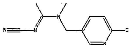
Acetamiprid
