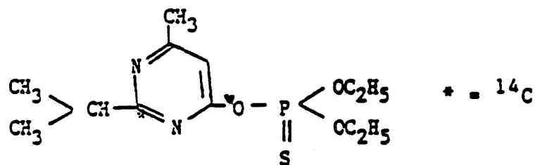
DIAZINON (G-24480)
