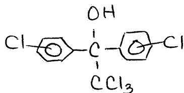
dicofol 1,1-bis(chlorophenyl)-2,2,2-trichloroethanol
