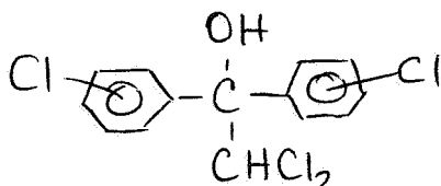
FW-152 1,1-bis(chlorophenyl)-2,2-dichloroethanol
