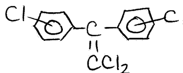
DDE 1,1-bis(chlorophenyl)-2,2-dichloroethylene
