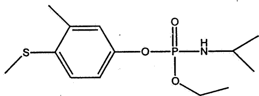
Fenamiphos
